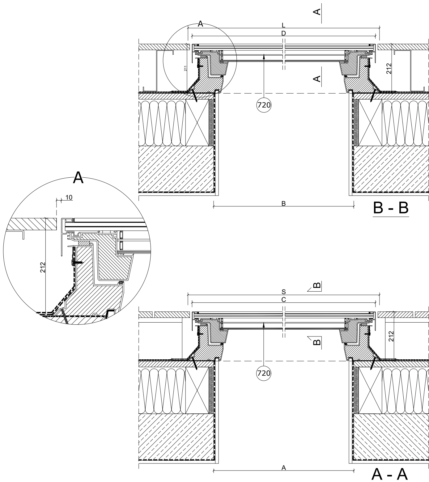
720-DXW DW6 świetlik do dachów płaskich, nieotwierany, szyba DW6
